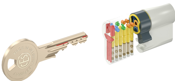
Afb.: Systeem 6 stiften
