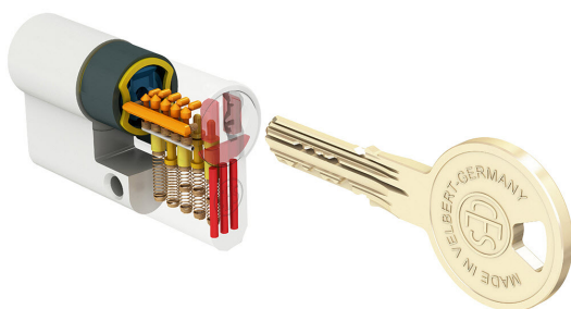
Afb.: System 5 stiften
